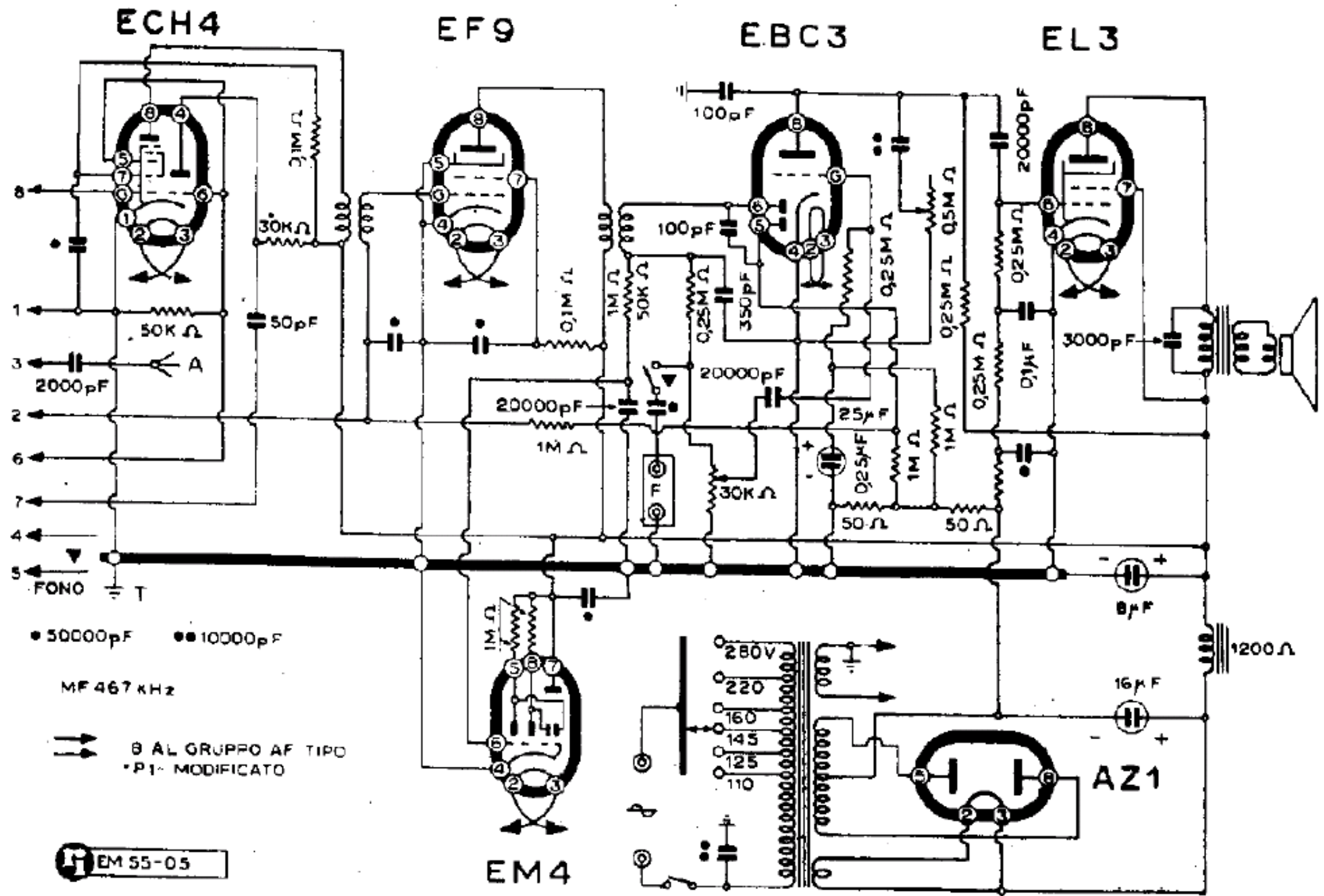
ELECTA RADIO - MOD. « ER 656-L »
